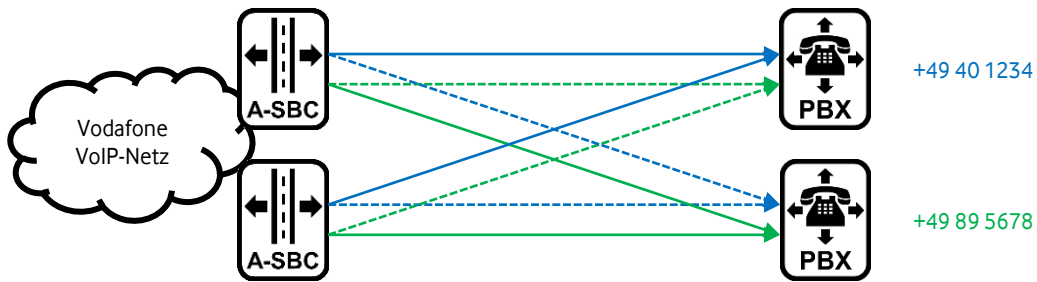
Abbildung 4: Rufnummernbasiertes Ausfallrouting
