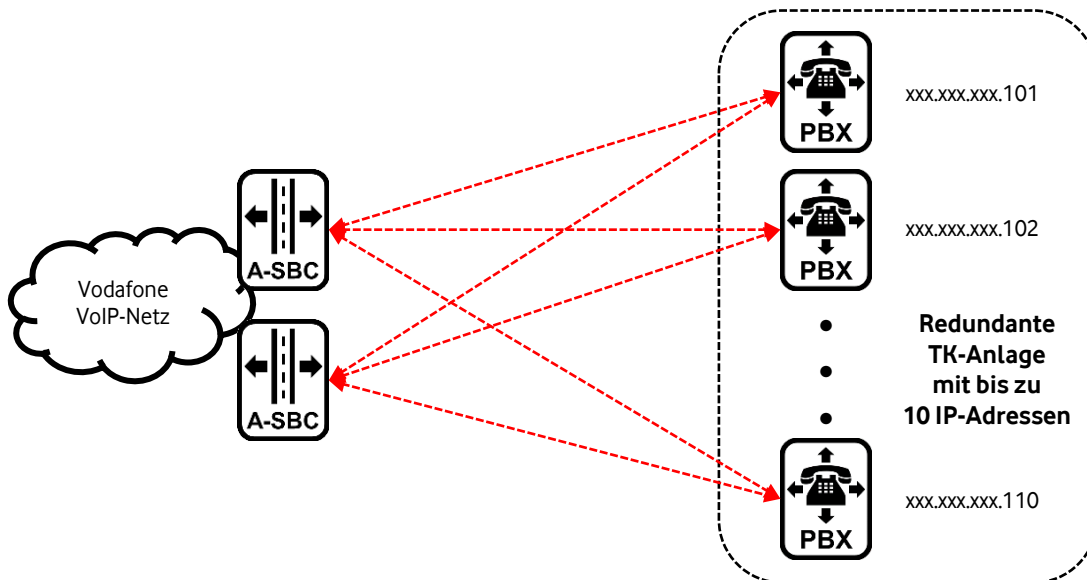
Abbildung 3: Redundante TK-Anlage
