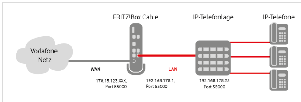
Abb. 27: Port Forwarding für SIP-Datenverkehr
