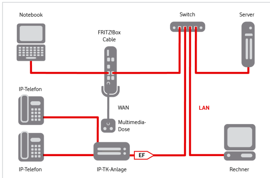
Abb. 26: Sprachpriorisierung, Anschaltung mit FRITZ!Box Cable
